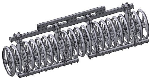
ЛДВ-6.20.000 Каток в сборе m = 620 кг.
