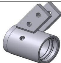
ЛДВ-6.16.250 Корпус m = 5,2 кг.
