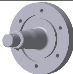
ЛДВ-4.00.201 Ось Материал: Ст45.m = 5,2 кг.
