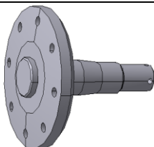
ЛДВ-6.16.205 Ось Материал: Ст45; m = 3,78 кг.
