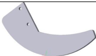
ЛДВ-4.12.001 Лыжа Материал: Ст45. m = 3,18 кг.
