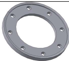
ЛДВ-6.16.002 Фланец Материал: Ст45; m = 1,1 кг.
