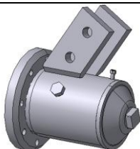
ЛДВ-6.16.200 Корпус в сборе m = 11,75 кг.
