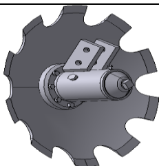
ЛДВ-6.16.000 Корпус с диском m = 20,75 кг.
