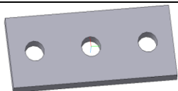
КШУ-8.00.033 Пластина Материал: Ст3пс, S=6мм. АхВ=145х60 мм., m = 0,4 кг.
